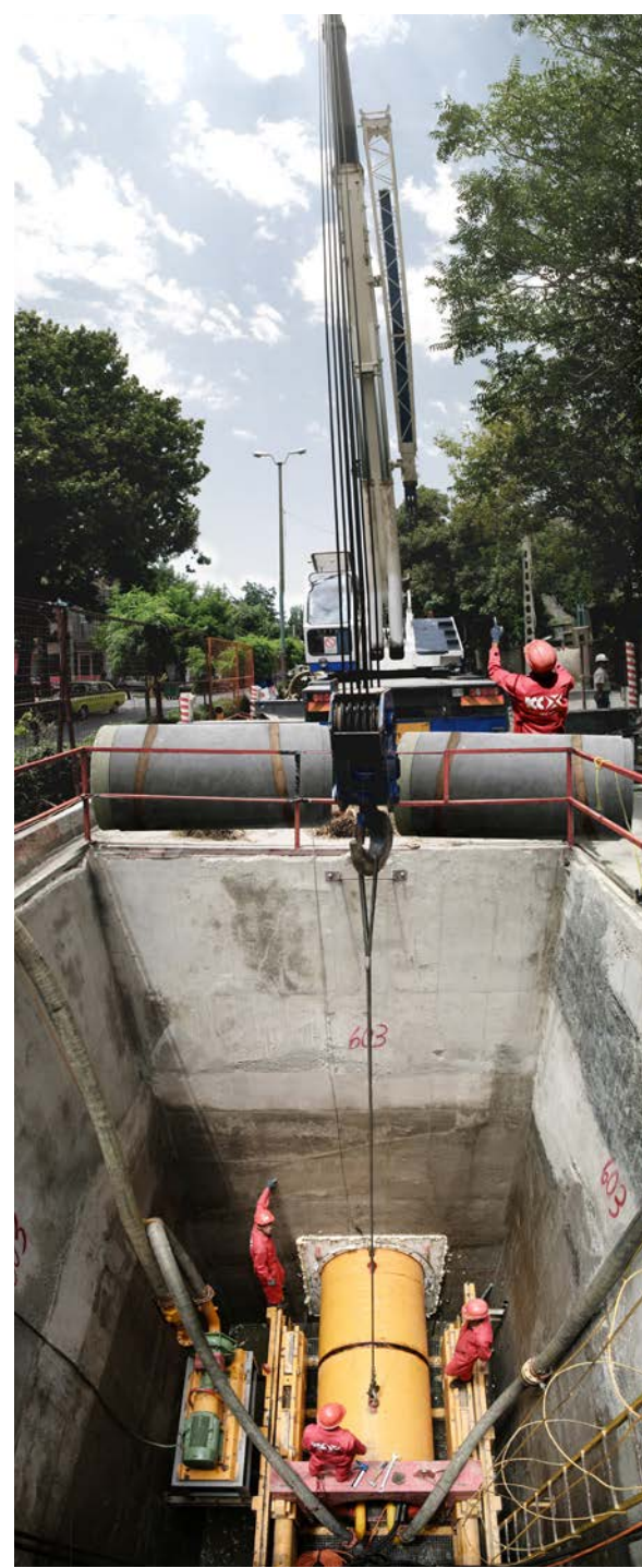
مشروع الصرف الصحي همدان على طريقة سحب الانبوب (منجز)
